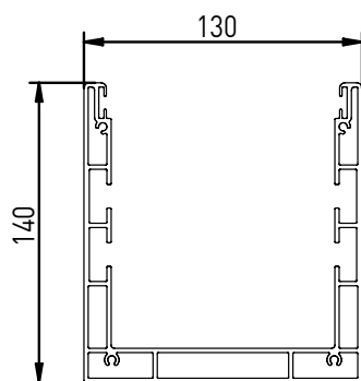
Viga frontal
