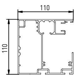
Guía
